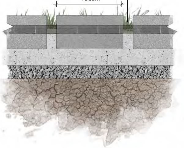
12 ábra: Áttört szegély metszet/oldalnézet
