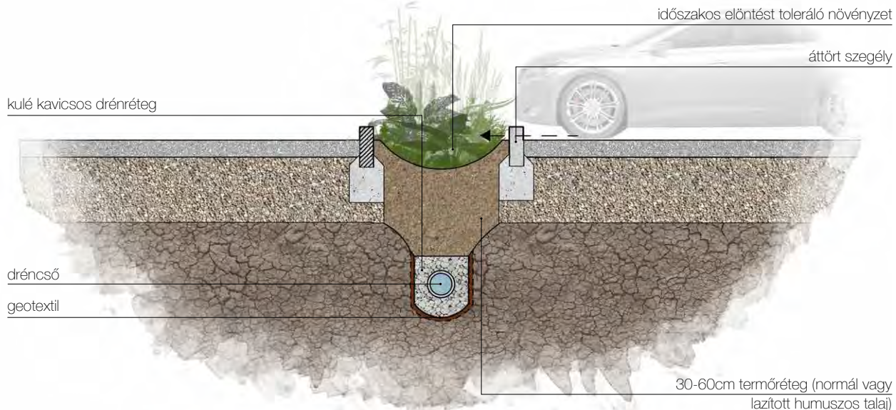
21. ábra: Esőkert részletrajz
